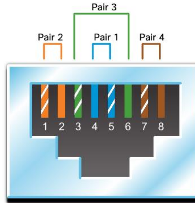
T568B
