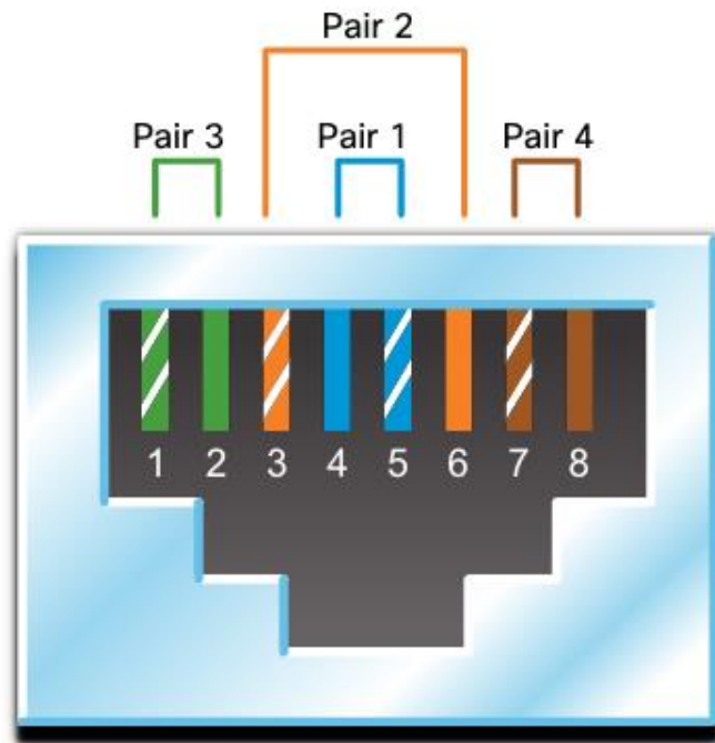
T568A
